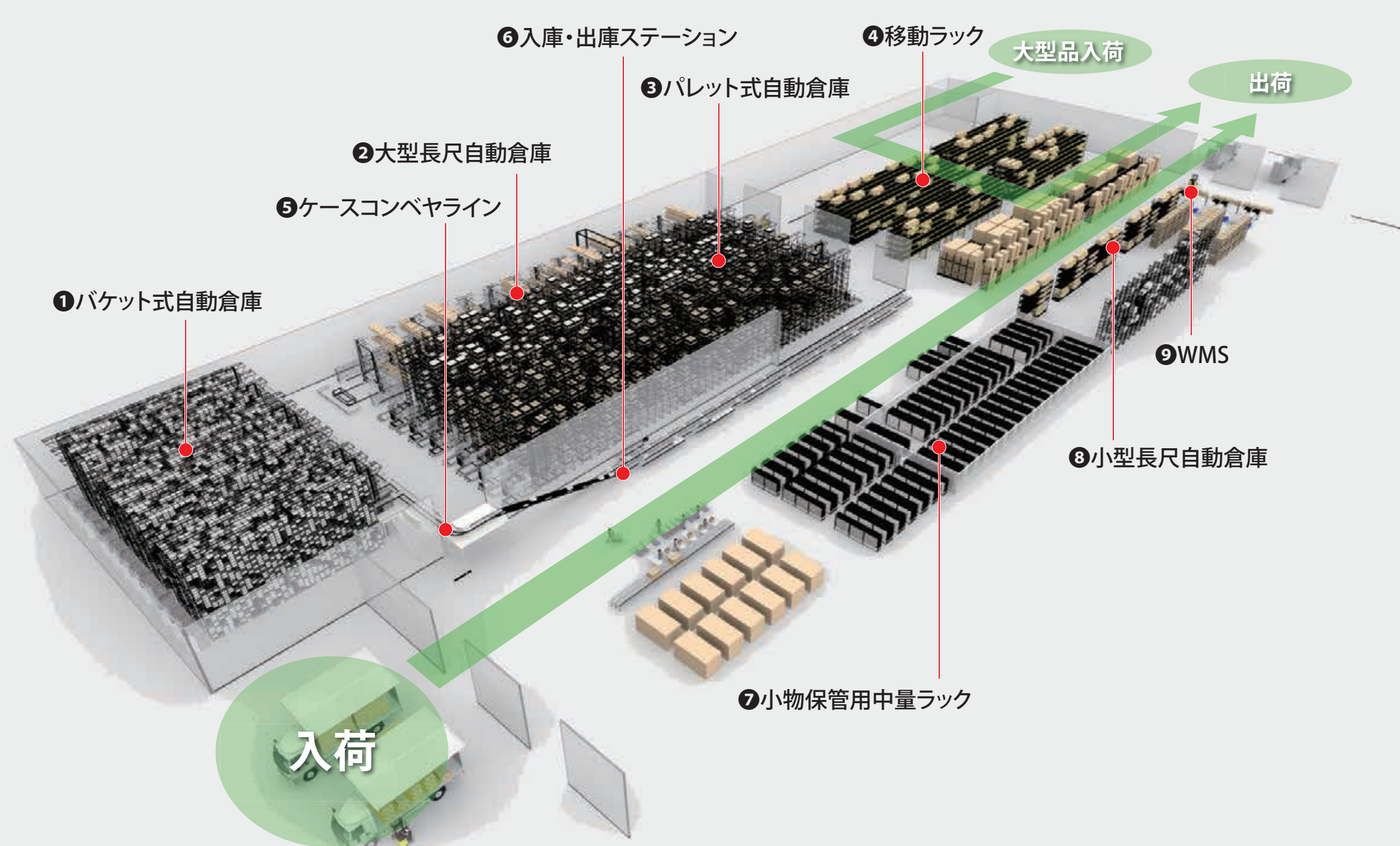
①バケット式自動倉庫 約8万点保管可能なバケット式自動倉庫を11台設置。
