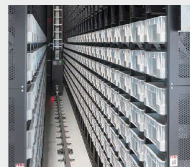
①バケット式自動倉庫 約8万点保管可能なバケット式自動倉庫を11台設置。
