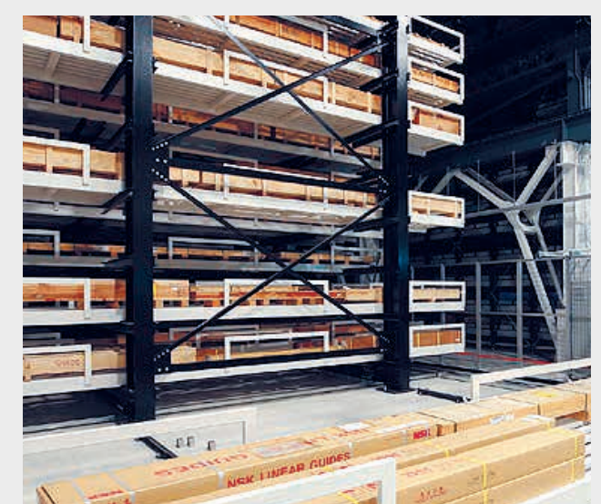
②大型長尺自動倉庫 オーダーメイド設計の倉庫であり、工作機械パーツのサイズに合わせて最大7mまでの収納が可能。
