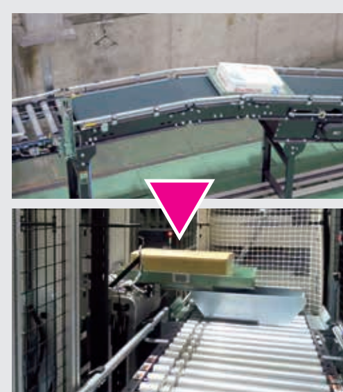
②入庫 登録完了後、コンベヤで搬送され、自動倉庫へ入庫。
